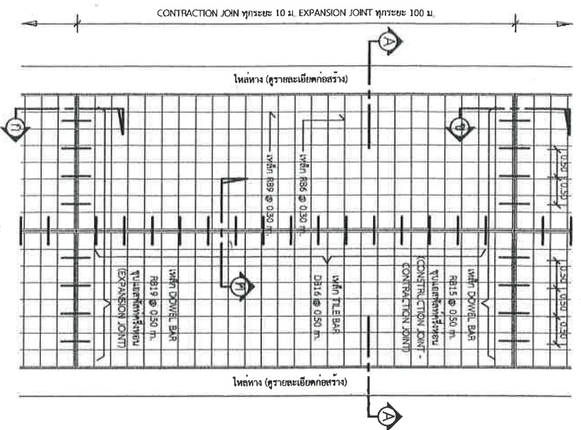
แบบแผนพื้นถาวร 1 : 75
