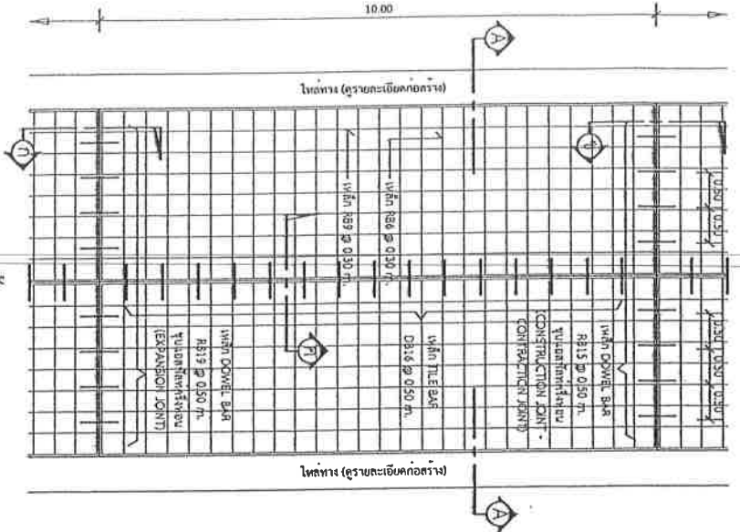
แปลนพื้นถนน 1 : 75
